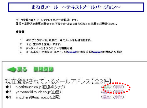
図 9 管理画面
